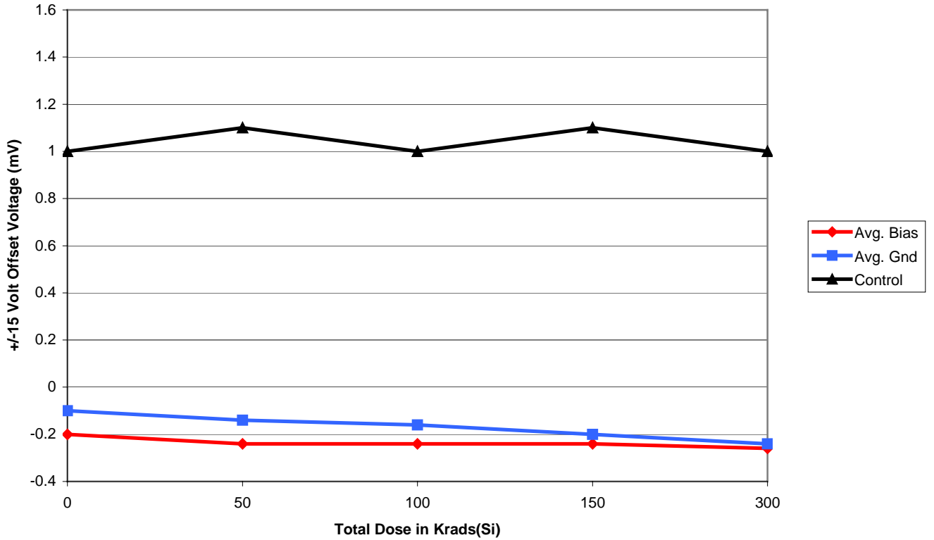
+/- 15 Volt Offset vs. Total Dose
